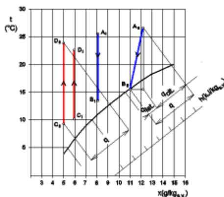
Obr.3 Znárodnění provozu výměníku ve stavu I a II v Mollierově i - x diagramu
