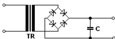
Obr.1 Usměrňovač zatížený kapacitou
