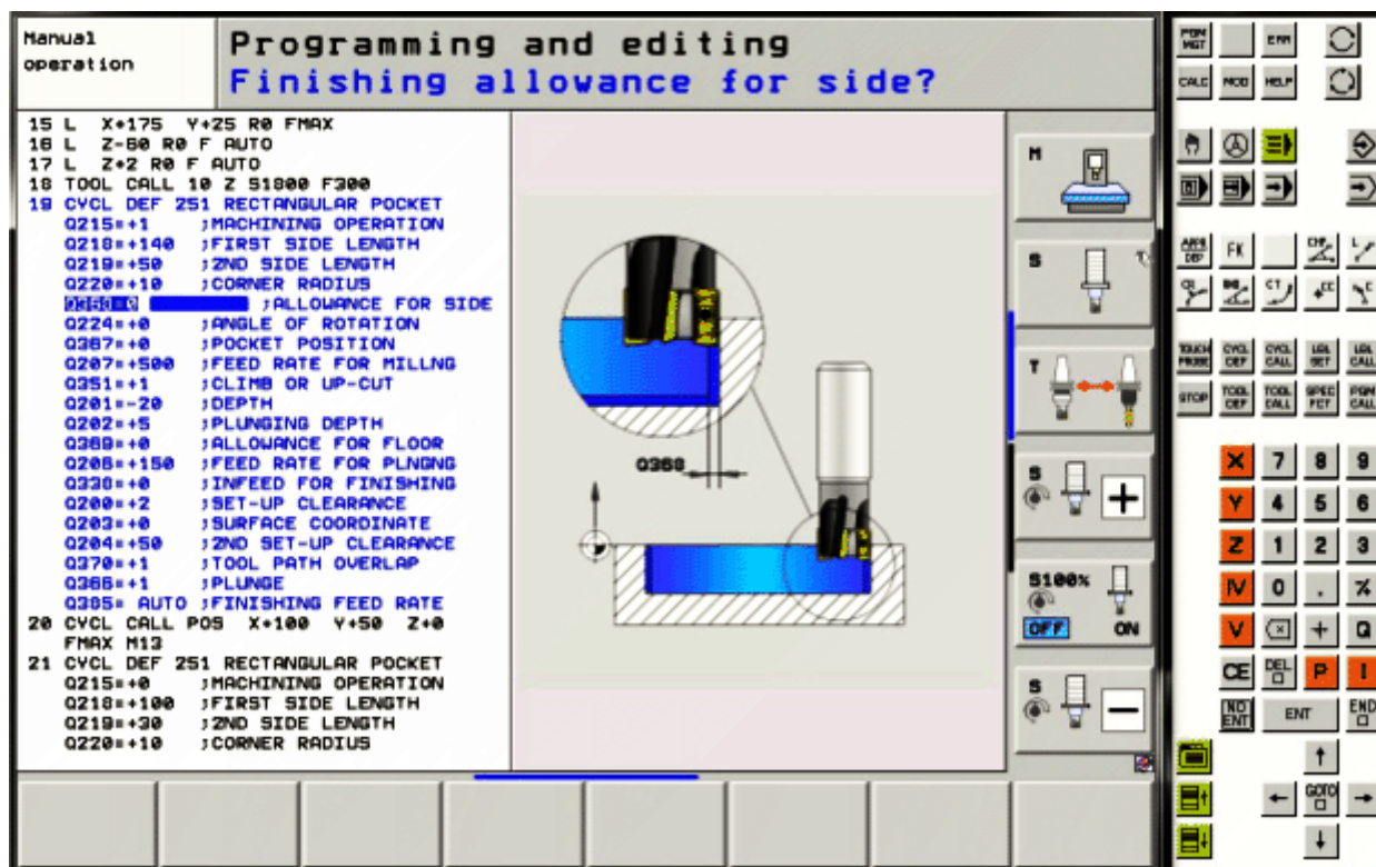
Obr.4 Dialogový obráběcí cyklus 251 umožňující programování prizmatického frézování a pomocí popisného dialogu programovat dráhu frézy s pomocí Q-parametrů [5]
