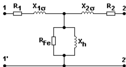
Obr.7 Náhradní schéma transformátoru
