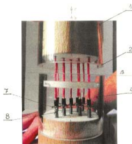
Obr.5 Zařízení při modelování namáhání TAH
