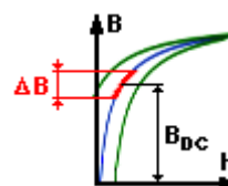
Obr.10 Magnetická indukce v jádru kompenzačního transformátoru
