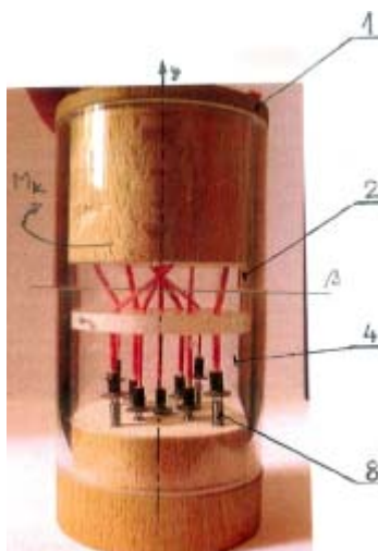
Obr.6 Zařízení při modelování namáhání KRUT
