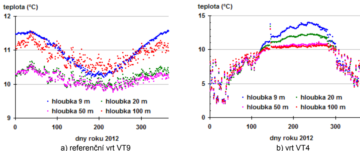
Graf 1 Průběh teploty horninového masivu ve 12:00 v různých hloubkách v roce 2012
