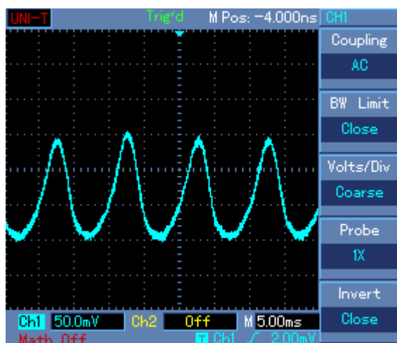
Obr.14 Oscilogram rozdílového napětí
