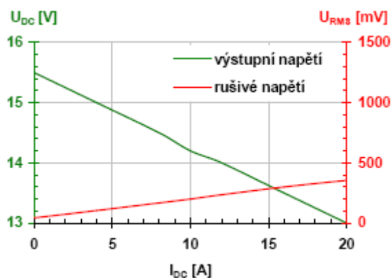
Obr.18 Závislost výstupního a rušivého napětí na velikosti odebíraného proudu
