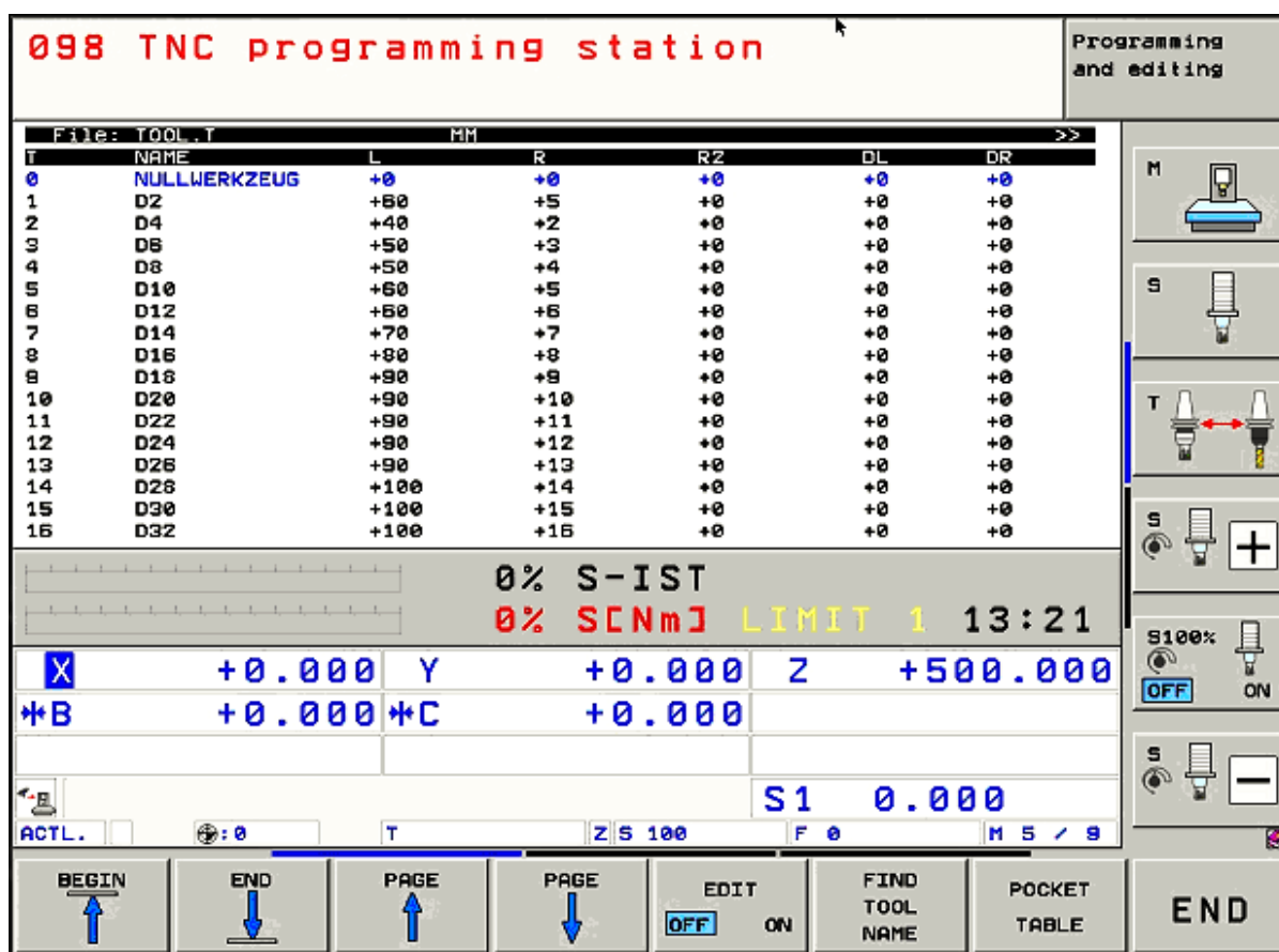
Obr.3 Zobrazení tabulky nástrojů (Tool Table) v řídicím systému HEIDENHAIN iTNC530 s možností editace korekcí řezných nástrojů na délku a průměr [5]
