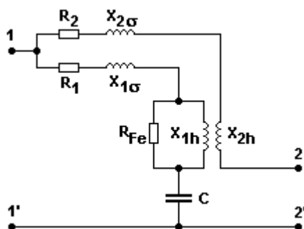
Obr.9 Náhradní schéma kompenzačního transformátoru
