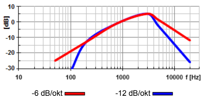
Obr.3 Frekvenční charakteristika komunikační linky
